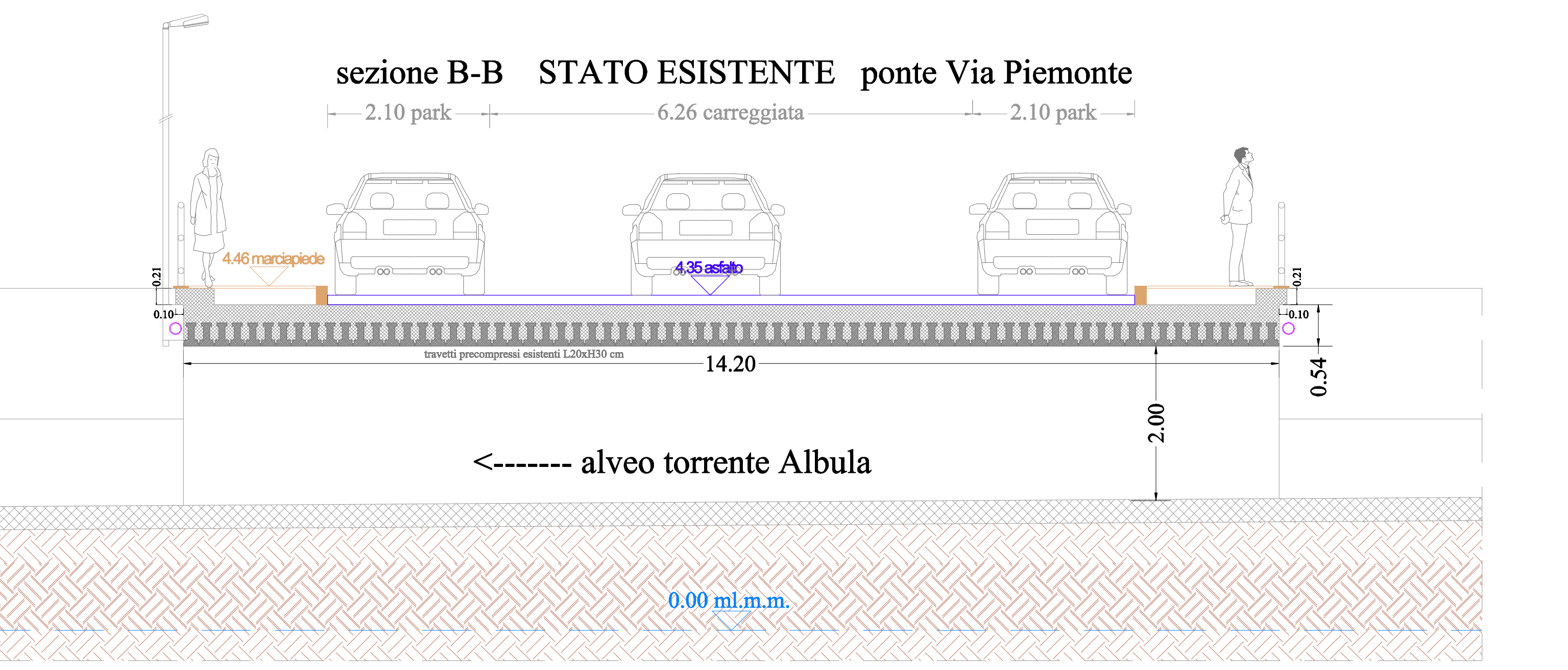
NOTA BENE: LE TUBAZIONI SPOSTATE DOVRANNO ESSERE OPPORTUNAMENTE ALLACCIATE ALLE LINEE ESISTENTI IN CORRISPONDENZA DELLE SPALLE IMPALCATO e SEZIONI STATO ESISTENTE SCALA 1:50
